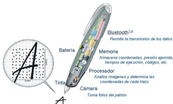
Fig. 2. Estructura del bolígrafo digital.
